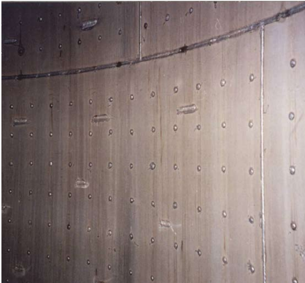
Acero 439A como revestimiento de un tacho de cocimiento de acero carbono en un ingenio después de 12 años de utilización
